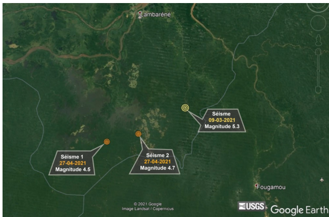
Localisation de l'épicentre du deuxième séisme (Source : USGS)
