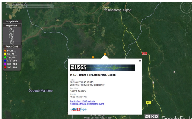
Localisation de l'épicentre du deuxième séisme (Source : USGS)
